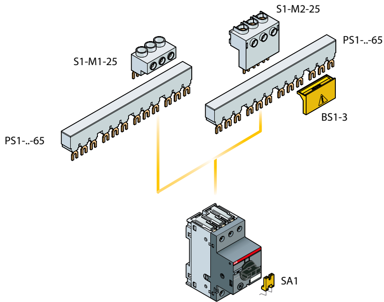
Busbar trifásico hasta 65 A
