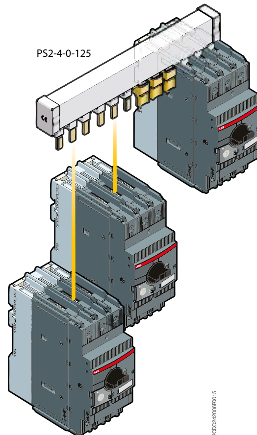
Busbar trifásico hasta 125 A
