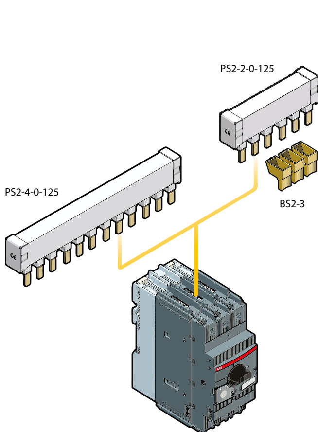
Busbar trifásico hasta 125 A
