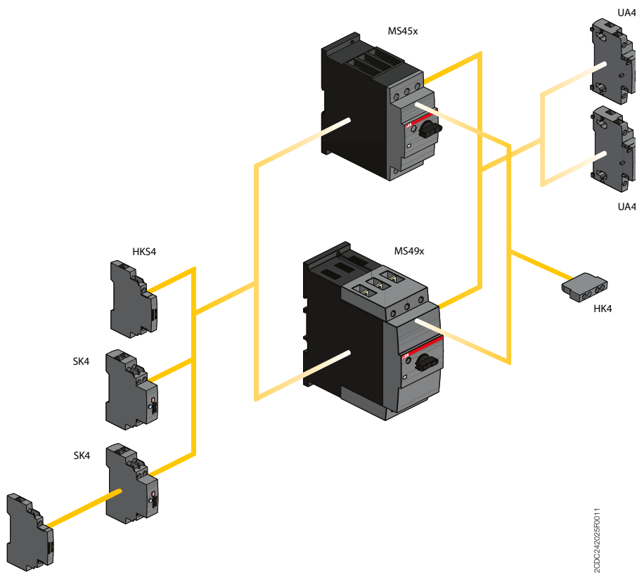
Guardamotor MS49x con accesorios
