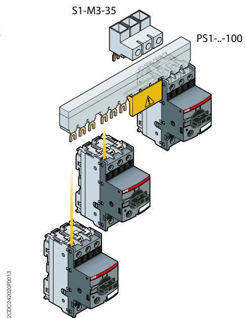
Busbar trifásico hasta 100 A
